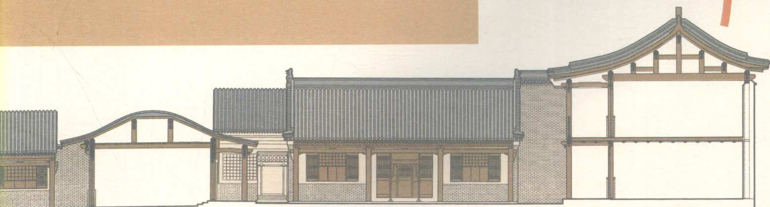
暖泉镇西古堡东楼房院第四进正房正立面复原图
