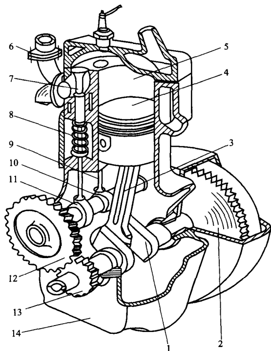
图 1-2 单缸内燃机
