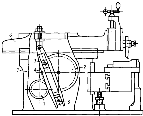
图 1-1 牛头刨床
