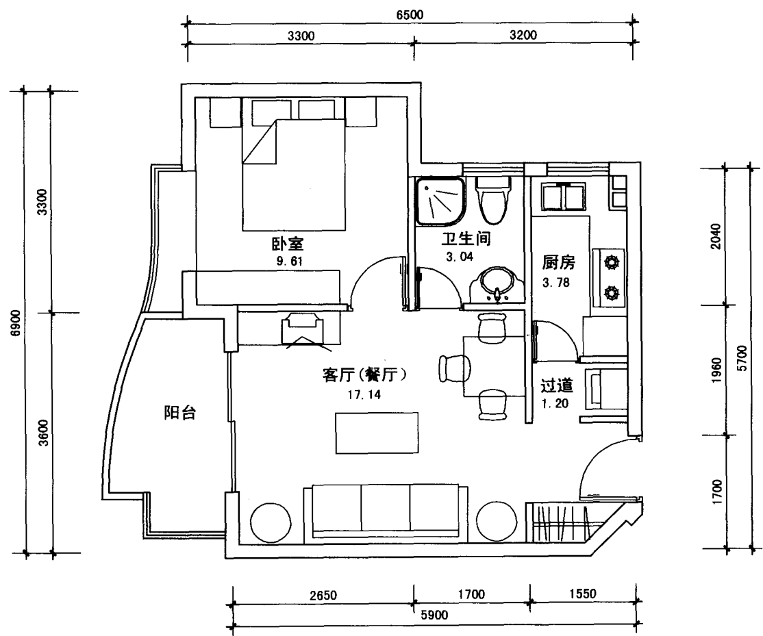
H2型户型平面图
