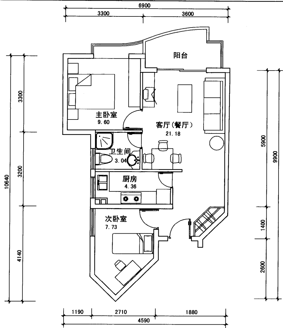
H2型户型平面图
