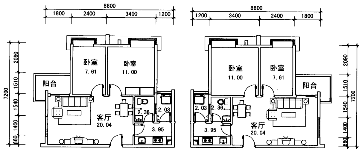
H1户型平面图
