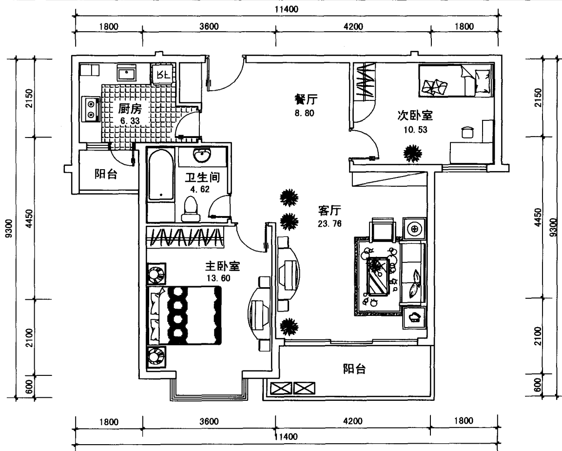
H3型户型平面图
