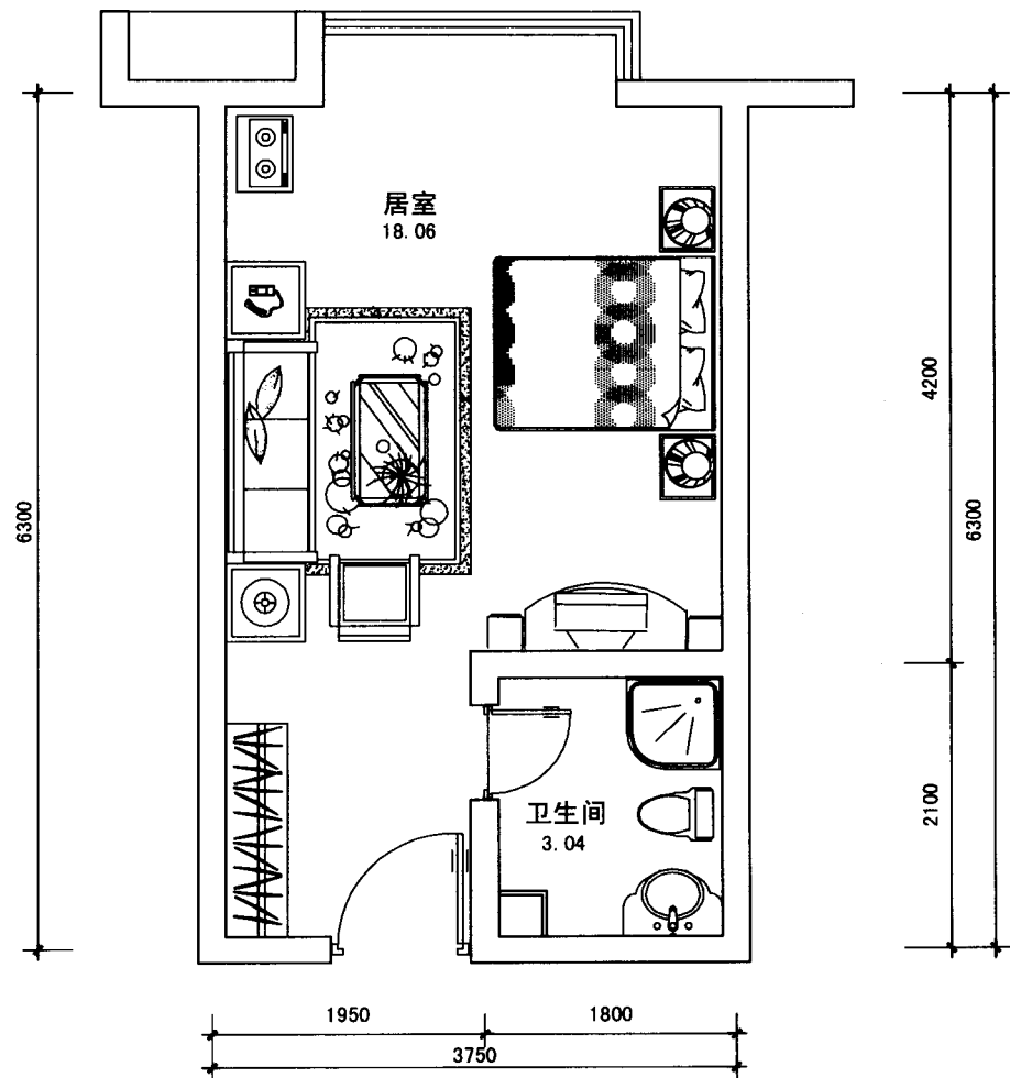
H2型户型平面图
