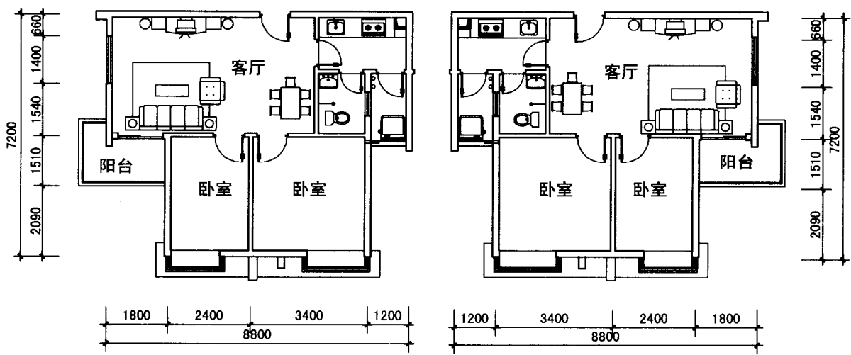
H1反型户型平面图
