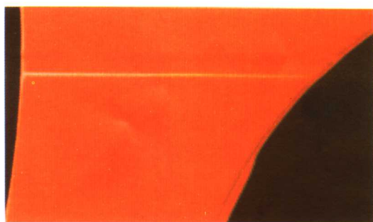
图9-42 流淌
