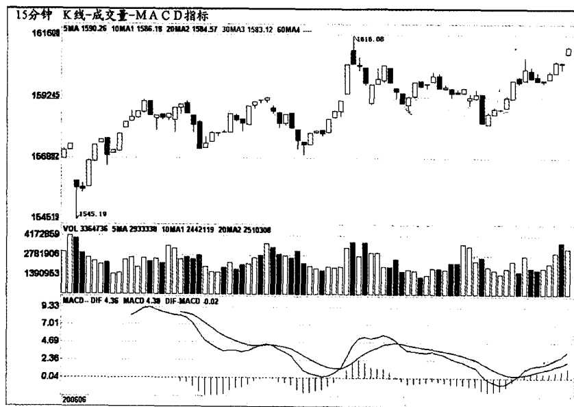
图 1-1 当日分时指数图
