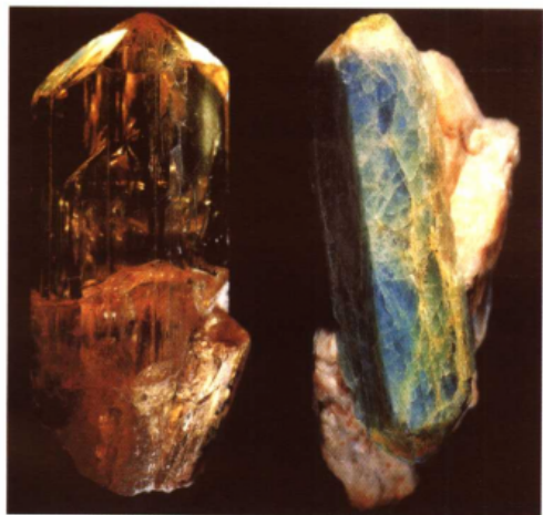
▲ 黄色、蓝色磷灰石晶体
