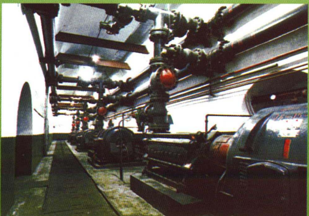
井下中央泵房
