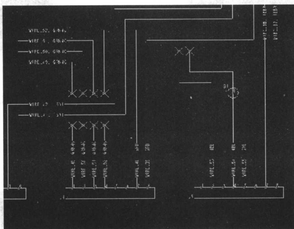
图 1-8 电器布线图
