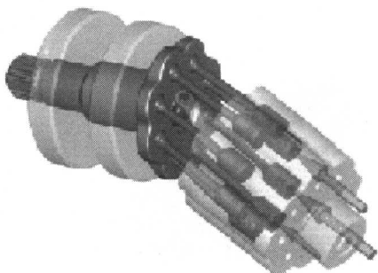
图 1-13 模型分析
