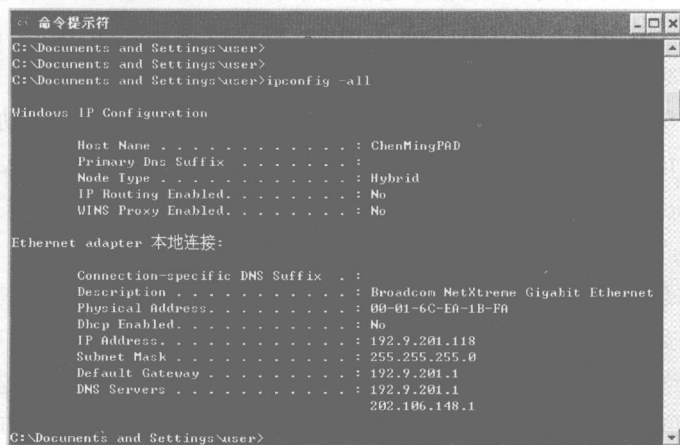
图 1-3 网络连接信息
