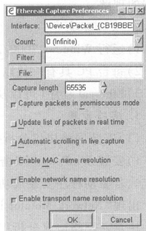
图 1-6 俘获分组配置界面
