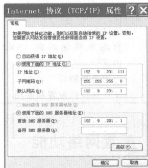
图 1-2 “Internet 协议属性”对话框
