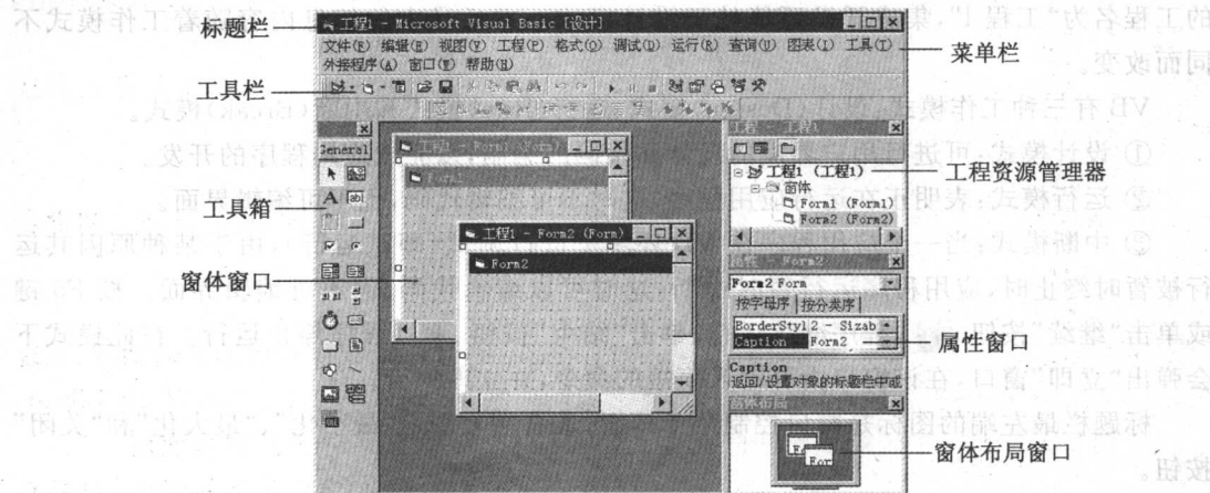
图 1-2 VB 6.0 应用程序集成开发环境
