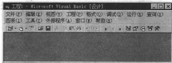
图 1-3 主窗口
