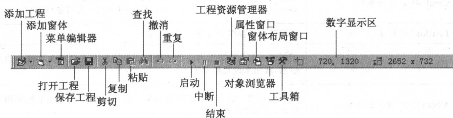
图 1-4 “标准”工具栏
