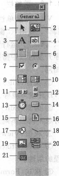
图 1-5 工具箱窗口
