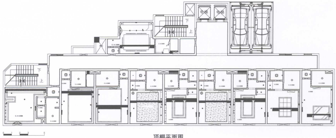
顶棚平面图
