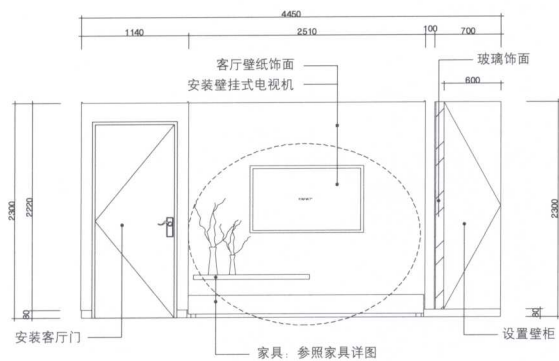
立面图 A, B
