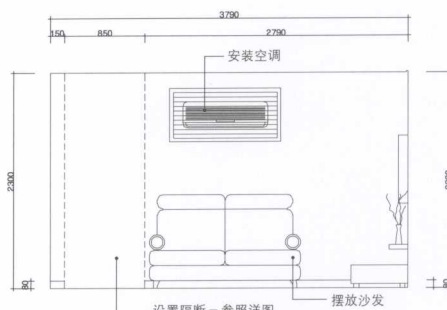
家具 - 正视图
