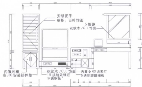
家具 - 正视图
