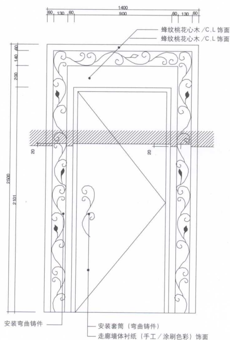
正视图
