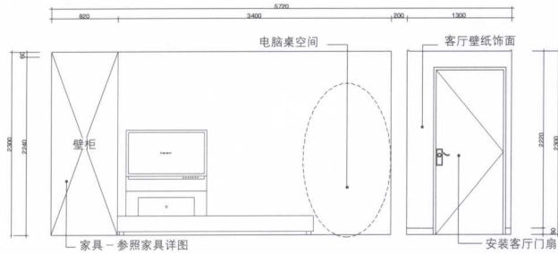
立面图 C,D
