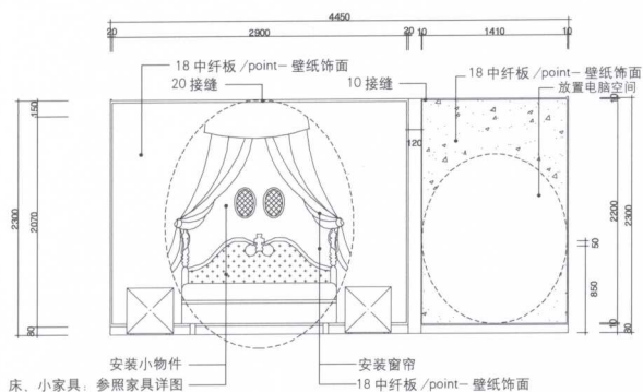
立面图 A, B
