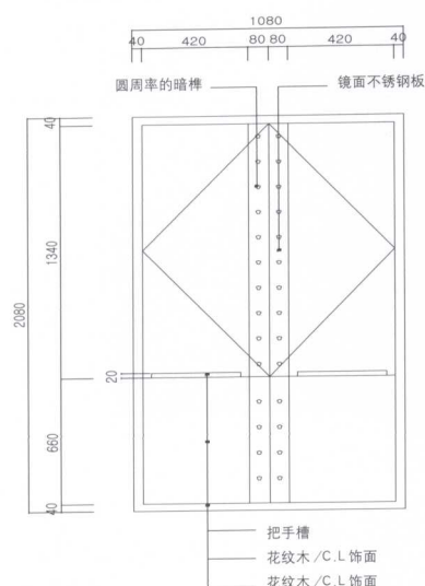
隔断门 - 正视图
