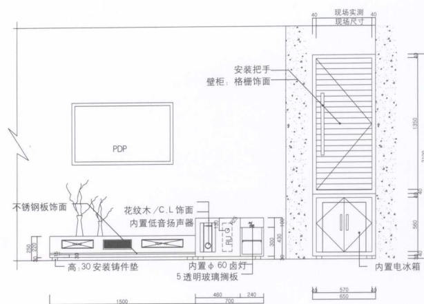
家具 - 正视图
