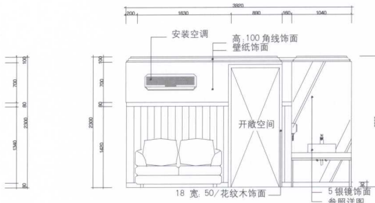
立面图 A,B
