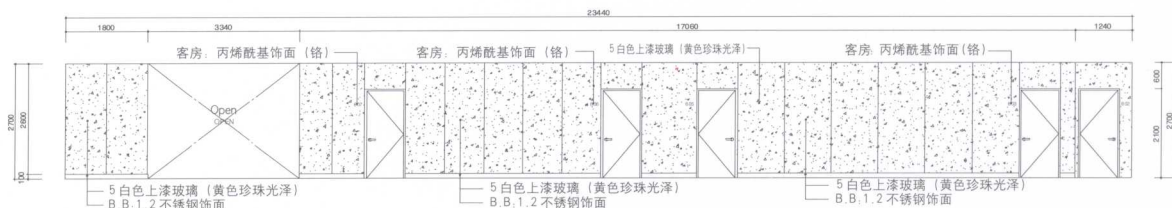
走廊—立面图 B
