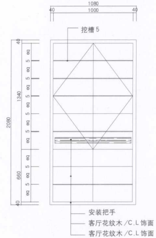
隔断门 - 正视图
