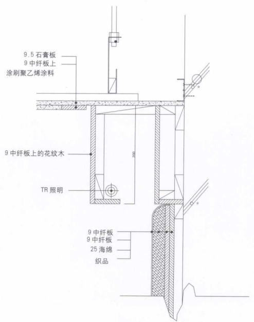
详图
