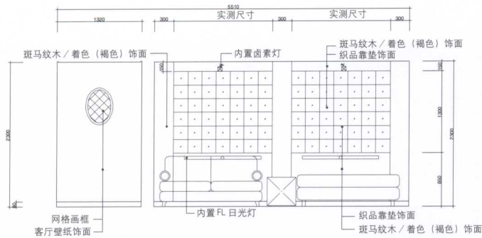
立面图 A,B
