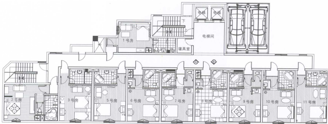
楼层平面图
