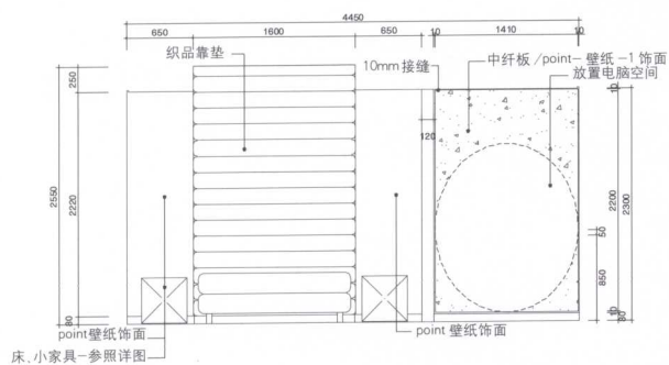
立面图 A, B
