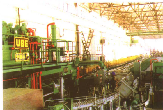
太原铝厂铝型材生产线
