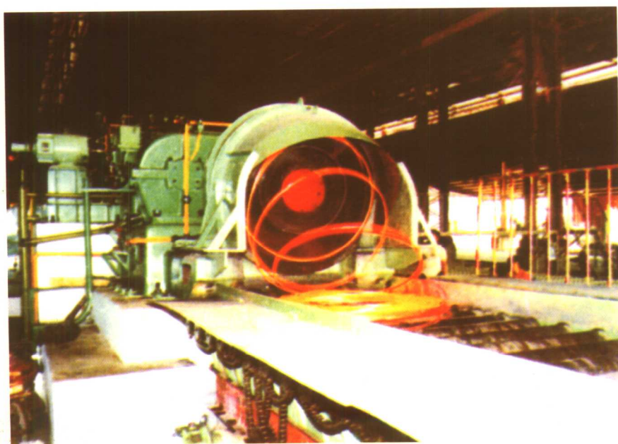
20世纪80年代初太原矿山机器厂生产的高速无扭线材精轧机
