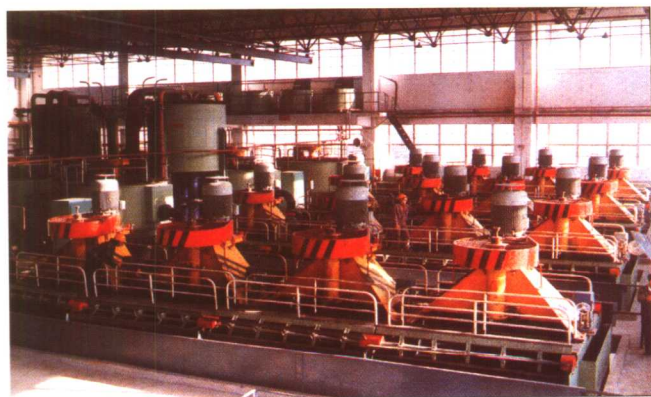
1994年建成的西山矿务局东曲矿选煤厂主洗车间
