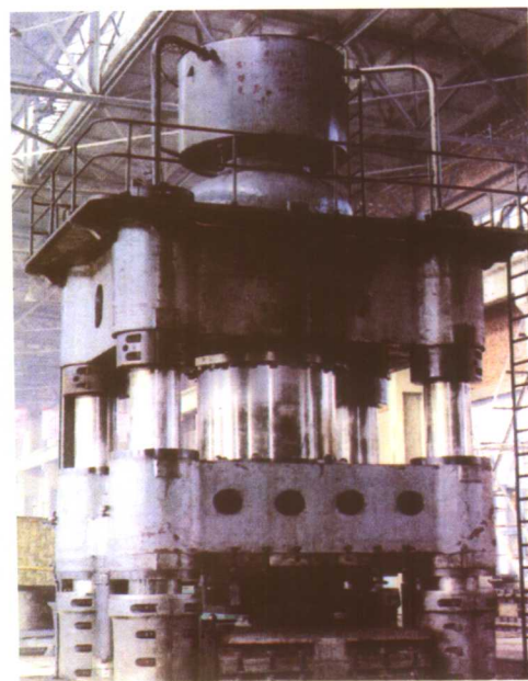
1982年太原重型机器厂制造的切边液压机
