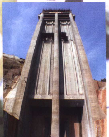
引水洞闸门
