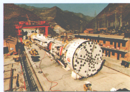
中国单线铁路最长的秦岭隧道 (18.4 公里)
