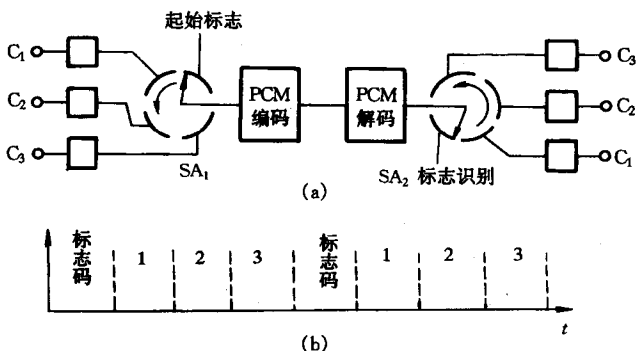
图 1-9 时分多路复用电路结构示意图
