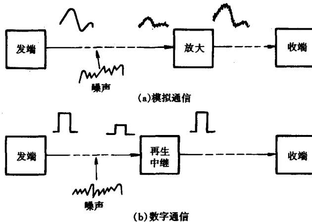
图 1-10 两类通信方式抗干扰性能比较
