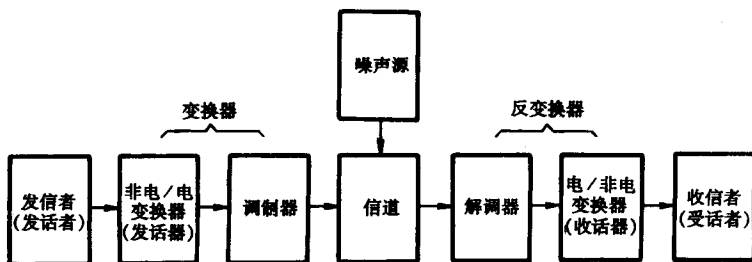
图 1-3 模拟通信系统实例
