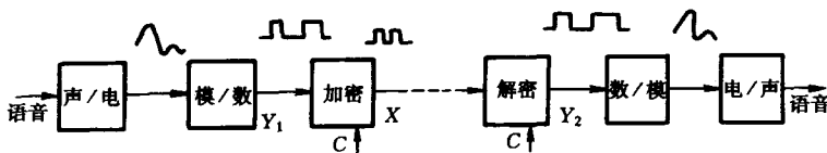
图 1-11 数字通信加密方法示意
