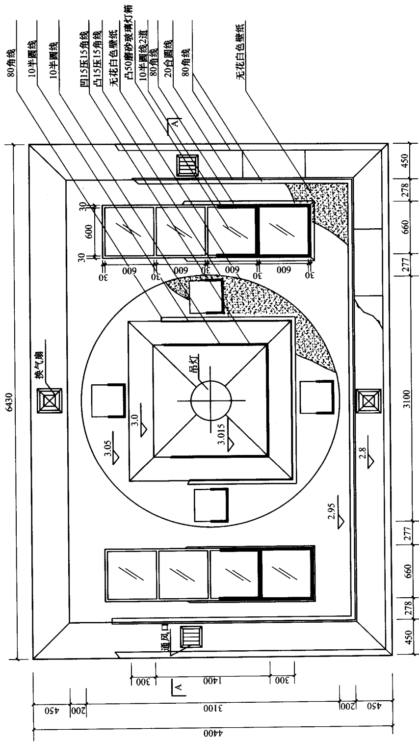
平面图
