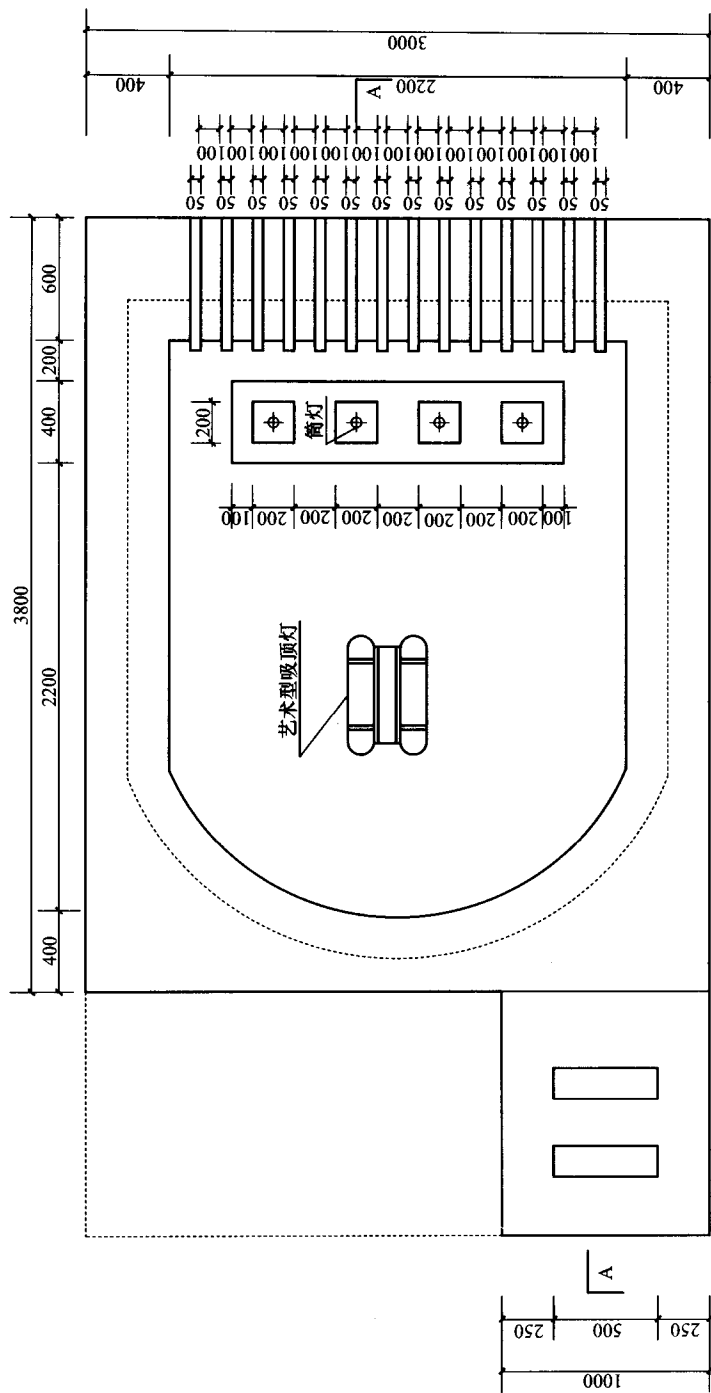
平面图
