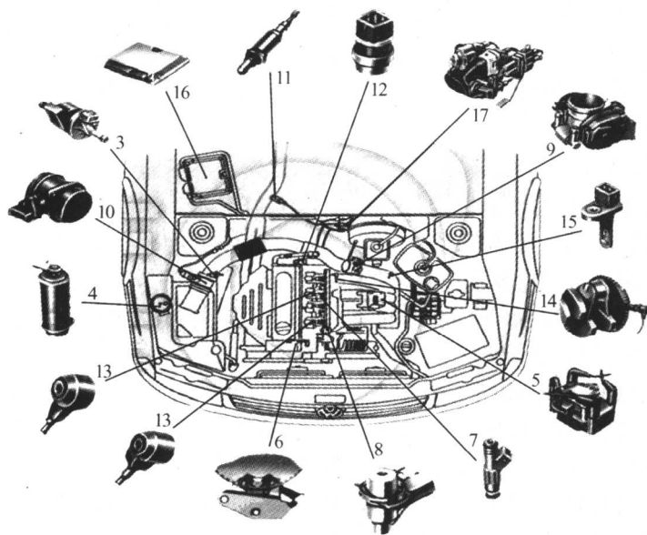
图 1-5 桑塔纳 2000GSi、3000 型轿车发动机电子控制系统控制部件的安装位置
