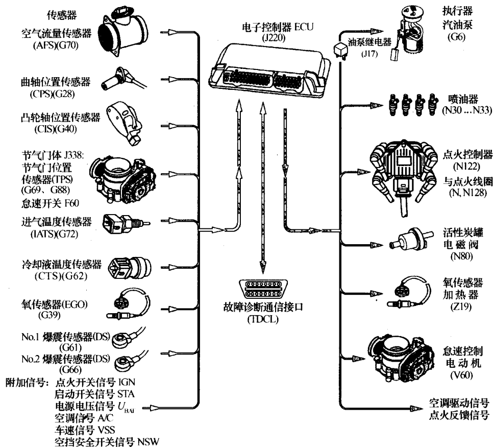
图 1-4 桑塔纳 2000GSi,3000 型轿车发动机电子控制系统控制部件的组成
