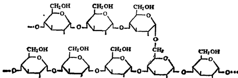
支链淀粉
