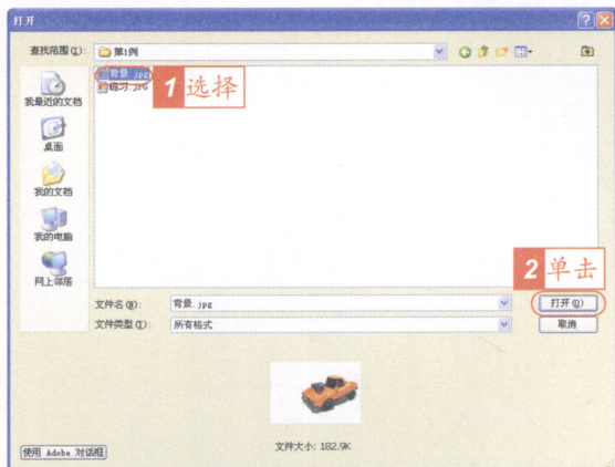
图1-1 “打开”对话框
