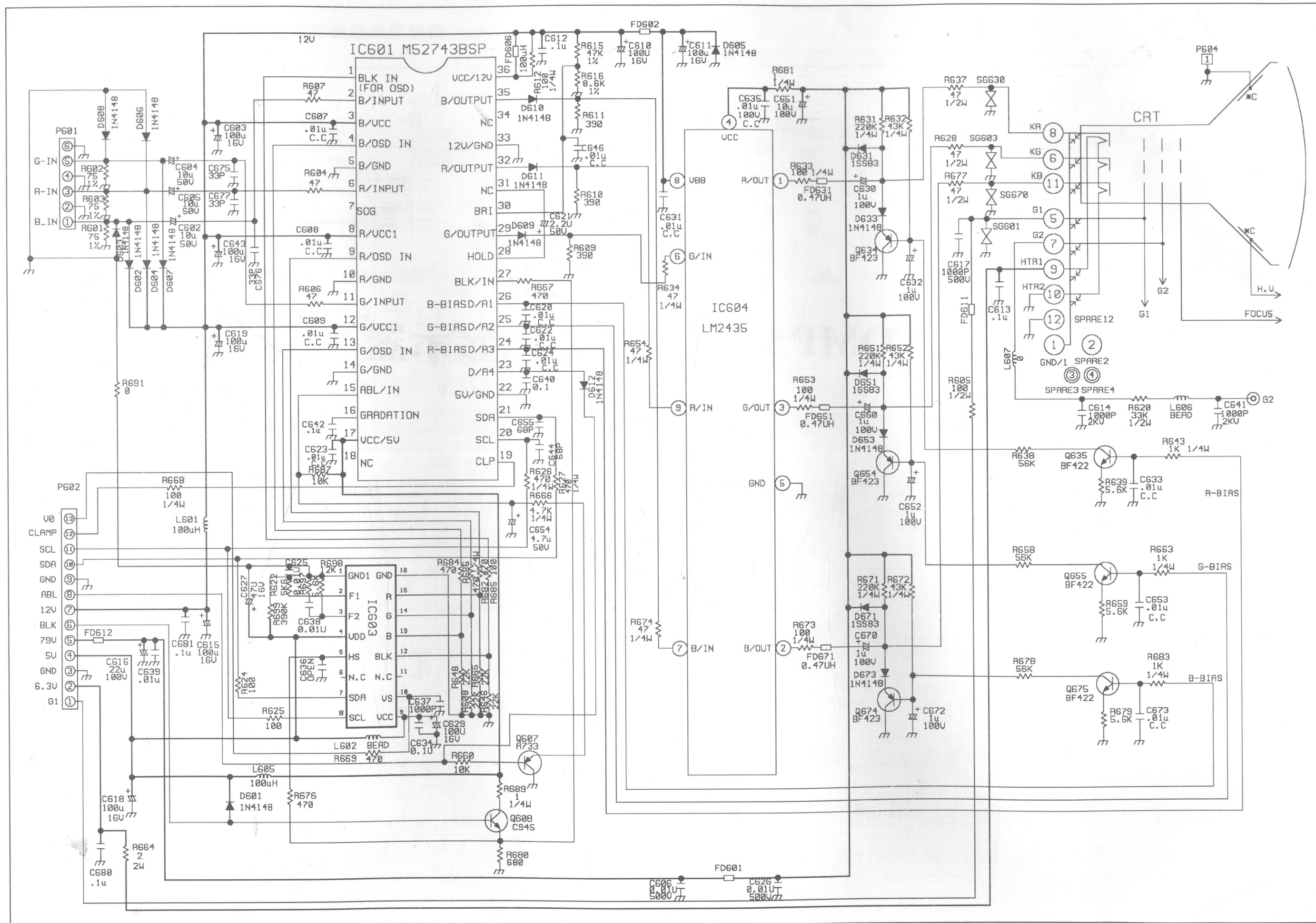
AOpen A90P 彩色显示器电路原理图(2/2)
