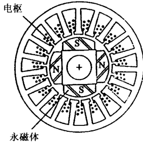
图 1.1 内转子结构
