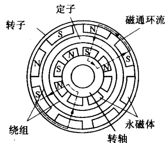
图 1.4 N-S 型双定转子式结构
