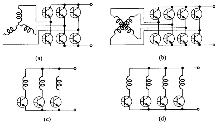
图 1.5 绕组的连接方式
