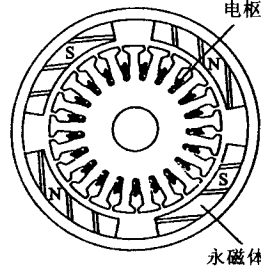
图 1.2 外转子结构
