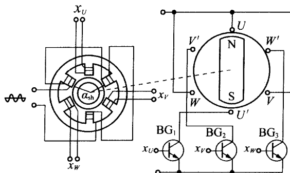
图 1.6 “三相星形非桥式”连接的电子换向(相)电路
