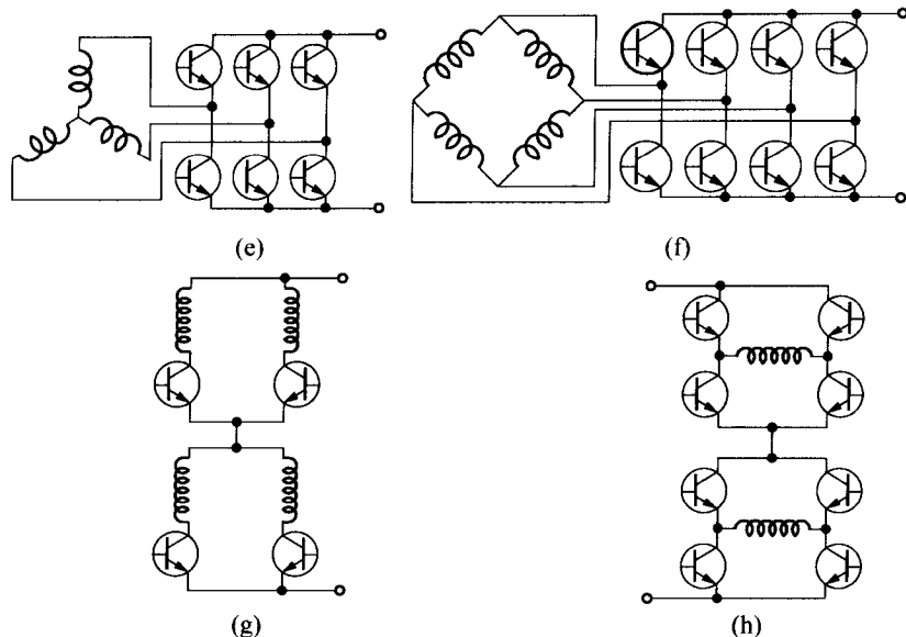
图 1.5 绕组的连接方式 (续)
