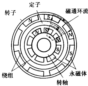
图 1.3 N-N 型双定转子式结构
