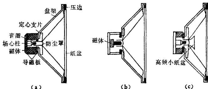
图 2-3 纸盆扬声器
