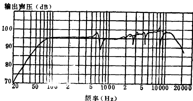
图 2-1 扬声器的频率特性曲线
