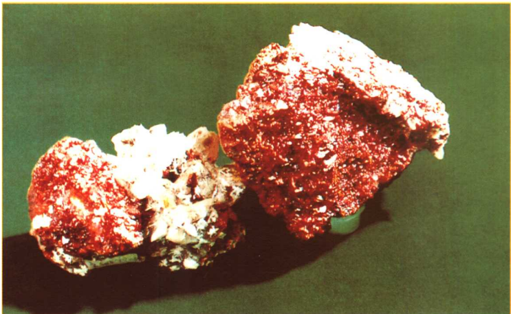
辰砂晶簇，万山特区产
