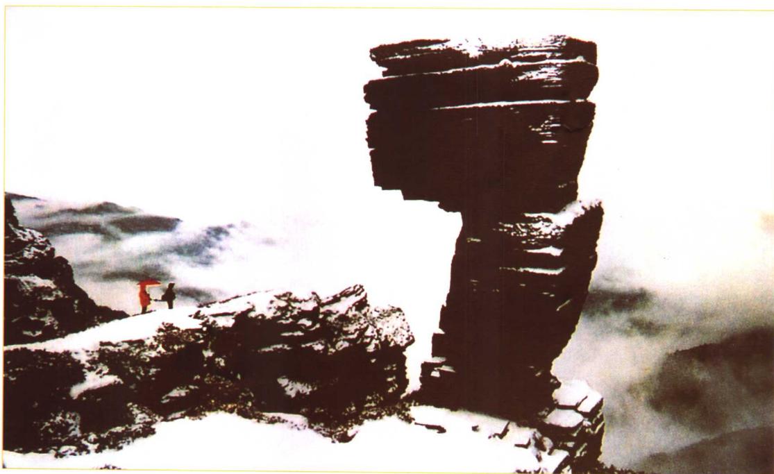
梵净山蘑菇石
