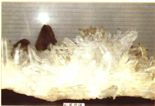
石英晶簇，万山特区岩屋坪产
