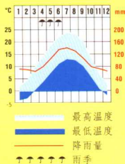
气候图 瑞士
