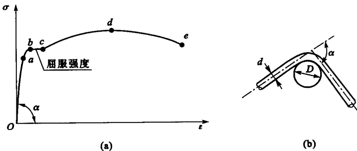
图 1.1 有明显屈服点钢筋的应力-应变曲线
