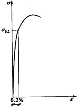
图 1.2 无明显屈服点钢筋的应力-应变曲线
