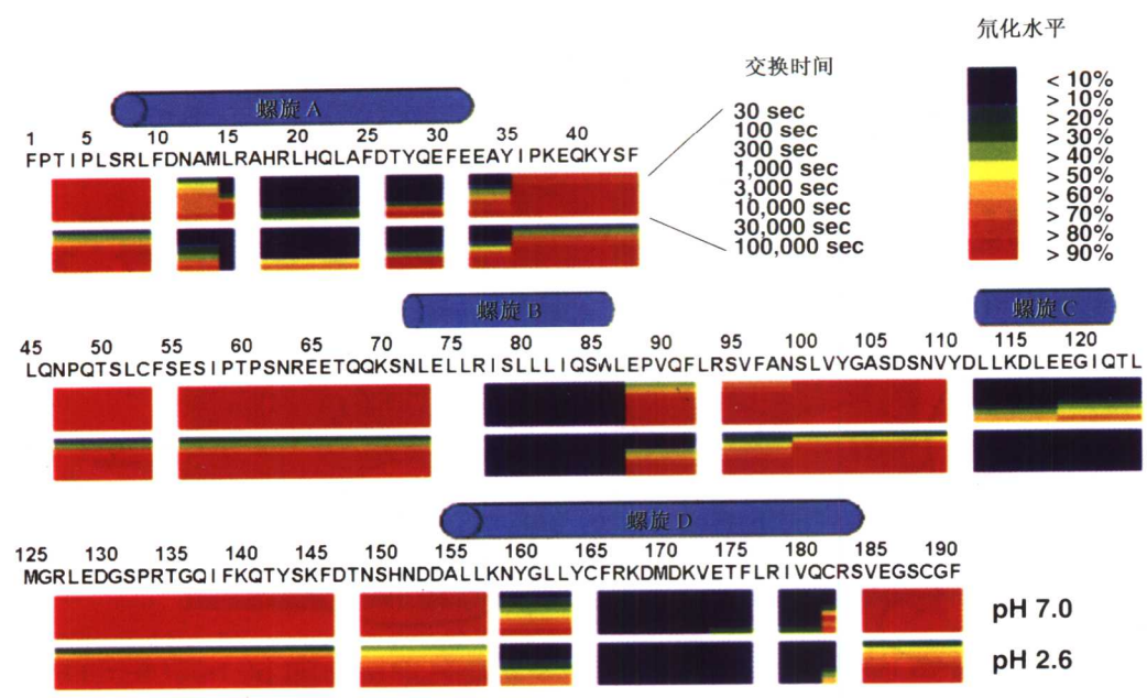
图 5.3 在 pH7.0 和 2.6 时人生长激素 (hGH) 的 H/D-Ex 分析 每个条块代表一种蛋白质产生的肽段。如右图所示, 每个条块由代表八个不同交换时间点的八个横条组成。在每个时间点每个肽的氘化水平用右上图所示的色彩表示。其中上排条块为 pH7.0 的交换情况, 而底排条块为 pH2.6 的交换情况。序列之上的淡蓝色圆柱形表示从 hGH (1HGU) 的 X 射线晶体结构中鉴定出的螺旋。含有最慢交换的酰胺氢用蓝色条带表示, 而含有最快交换的酰胺氢用红色条带表示。经 Hamuro 允许, 对图有改动 (Hamuro et al., 2003a)
