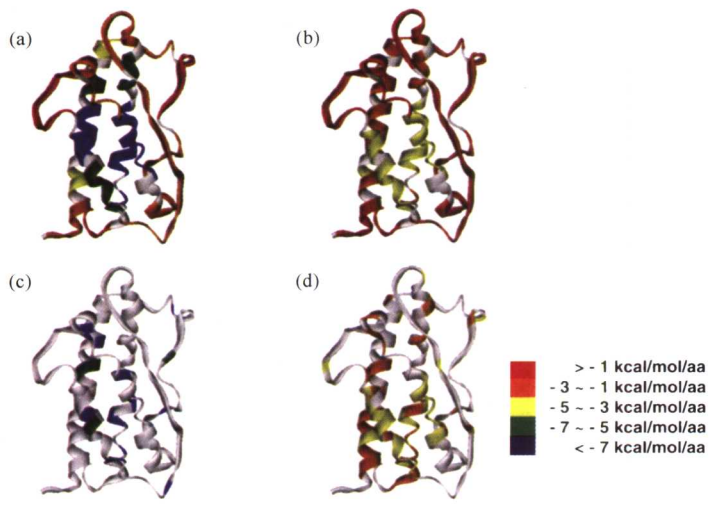
图 5.4 MS 和 NMR 测定的自由能随 hGH 折叠的变化 (a) 为 pH7.0 时 MS 的测定结果。(b) 为 pH2.6 时 MS 的测定结果。(c) 为 pH7.0 时 NMR 的测定结果。(d) 为 pH2.6 时 NMR 的测定结果。按照右下所示的图例, 将折叠自由能以彩色片段形式绘制在 X 射线结构图上 (1HGU)。灰色表示所用的方法未能分析出的残基。经 Hamuro 允许, 对图有改动 (Hamuro et al., 2003a)
