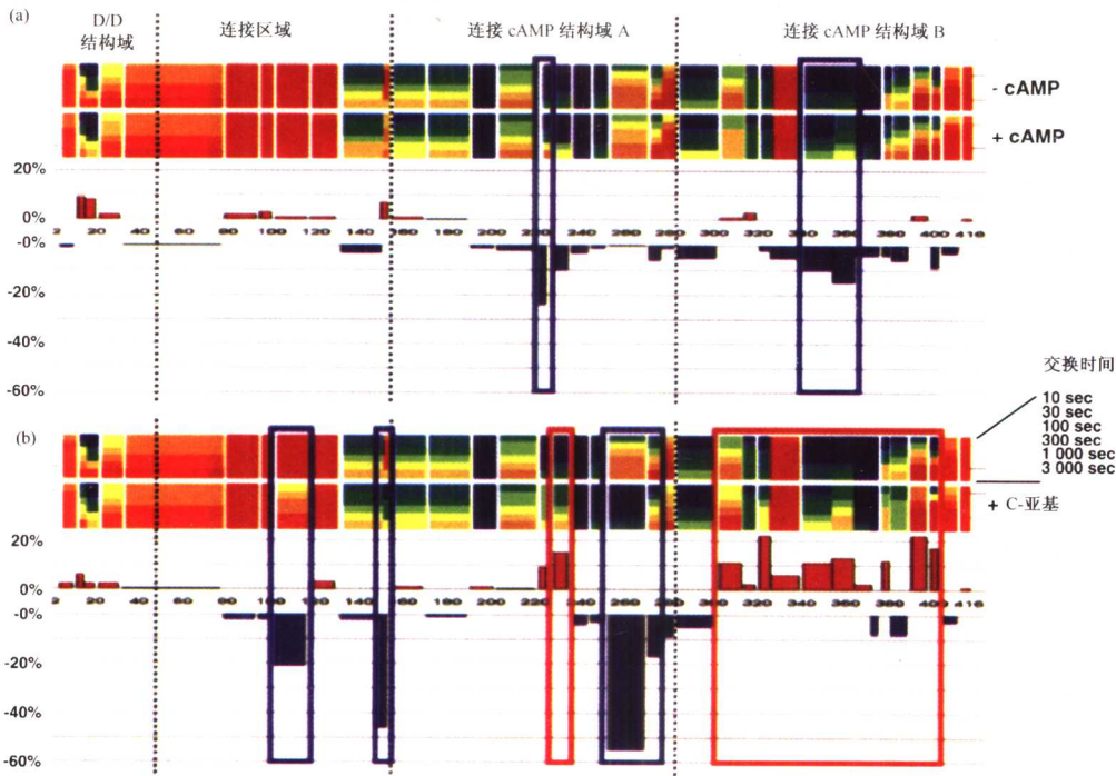
图 5.5 (a) 脱辅基 RII 的 H/D-Ex 结果 (上); 与 cAMP 结合的 RII 的 H/D-Ex 结果 (中); 结合 / 未结合 cAMP 的氧化水平的平均差异 (底)
