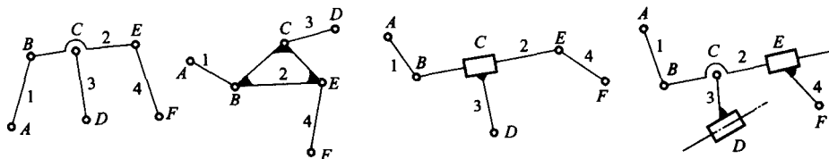
图 2-9 Ⅲ级杆组
