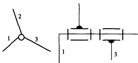
图 2-1 复合铰链
