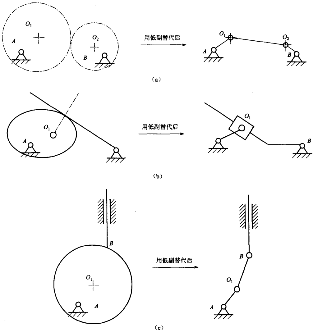
图 2-7 高副低代的常见情况
