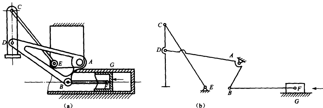
图 2-12 翻台机构
