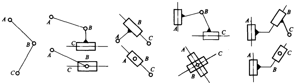
图 2-8 Ⅱ级组
