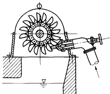
图 1-3 水斗式水轮机
