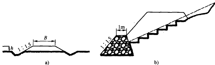
图 1-1-1 路基或填方路堤横断面图
