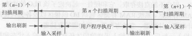
图 1-2 PLC 工作过程
