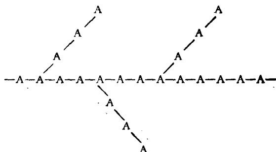
支链型
