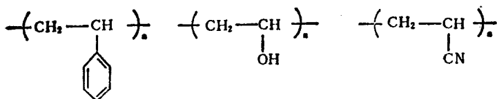
聚乙烯醇
