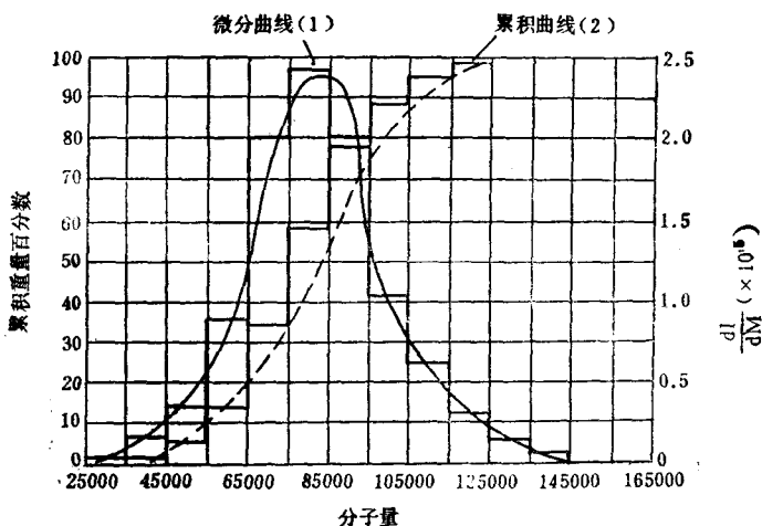
图 1-1 某一聚苯乙烯试样累积重量分布曲线和微分重量分布曲线
