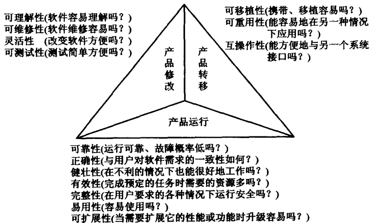
图 1-1 软件产品的质量特性图示
