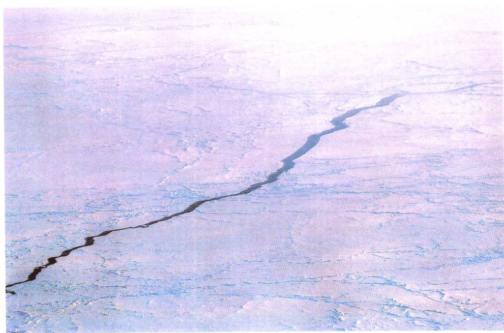
从数千米高空中拍到的北冰洋冰缝
