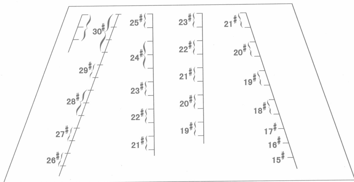
402型扬琴琴弦序列图
