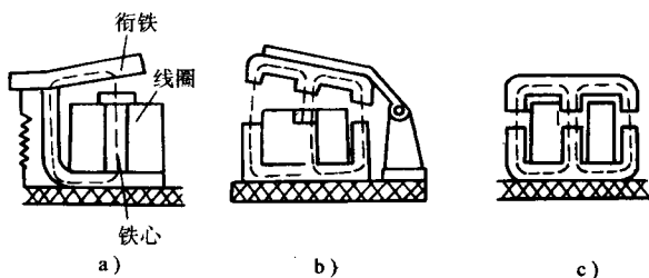
图 1-2 接触器电磁系统的结构图
