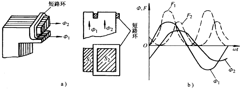
图 1-13 交流接触器铁心的短路环
