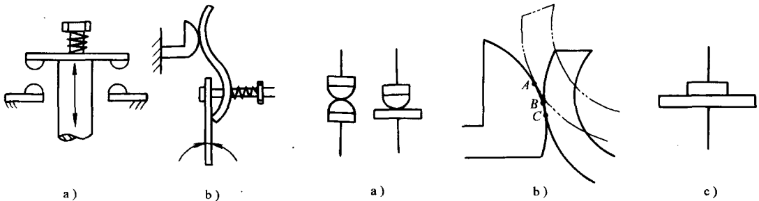
图 1-6 触头结构形式图
