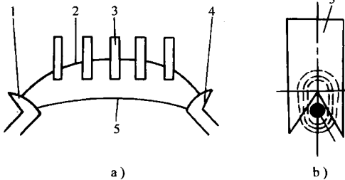
图 1-8 灭弧栅灭弧原理
