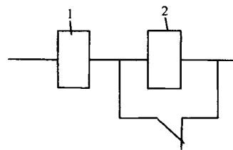
图 1-16 直流接触器双绕组线圈接线图
