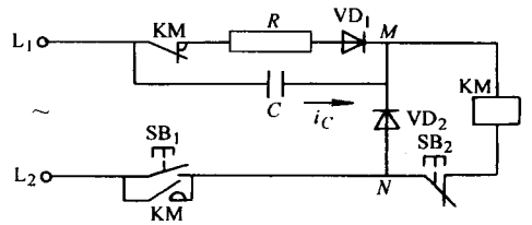
图 1-14 交流接触器无声节电装置线路
