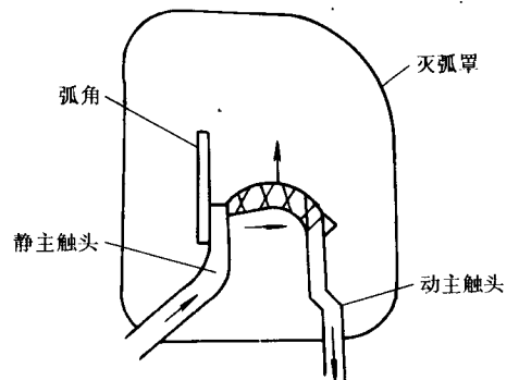
图 1-10 多纵缝灭弧装置
