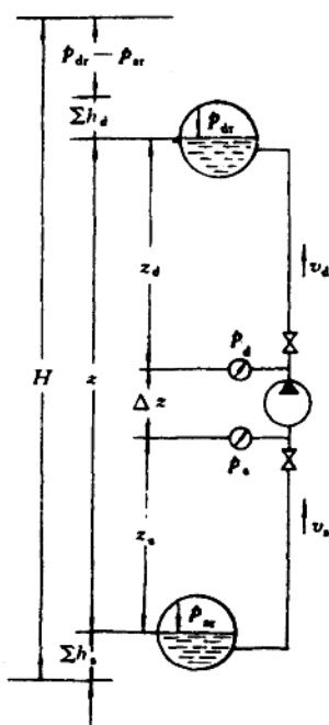
图 0-1 泵装置简图
