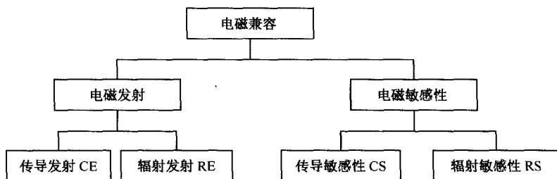
图 1-1 电磁兼容性的研究
