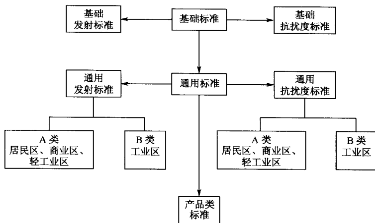
图 1-2 国际电磁兼容标准体系
