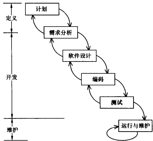
图 1.1 软件生命周期的瀑布模型
