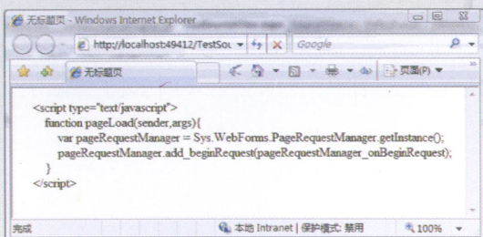
代码显示控件
