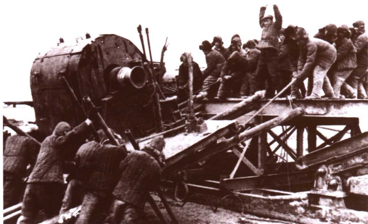
1960年4月2日，1205钻井队在大庆会战中采用“卸车坑”的方法将钻机从火车上卸下来。
