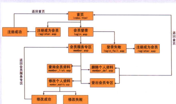
会员服务系统结构图
