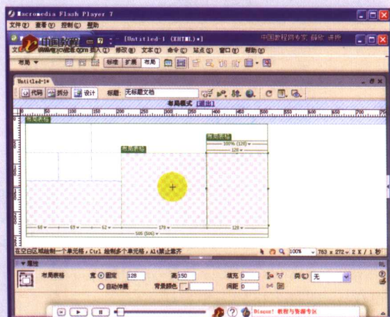
布局
