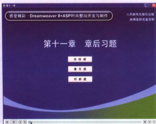
交互控制
