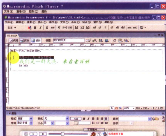
文本控制
