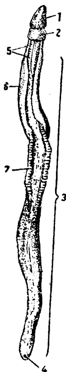
圖 2. 柱頭蟲(背面全圖)
