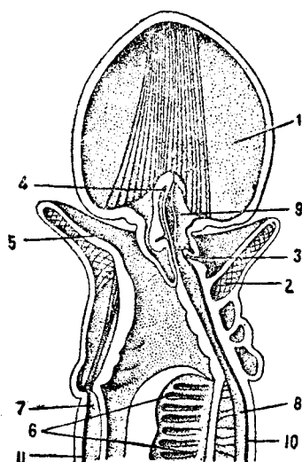
圖 3. 柱頭蟲頭部矢切面的模式圖。圖的左部為腹面, 右部為背面。
