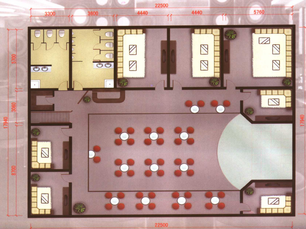
舞厅一楼、二楼平面布置效果图
