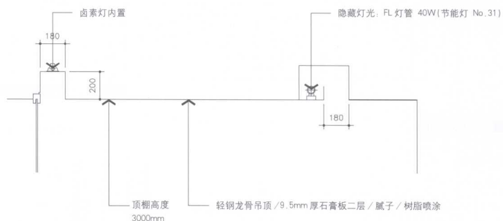
顶棚局部一剖面图 C、D
