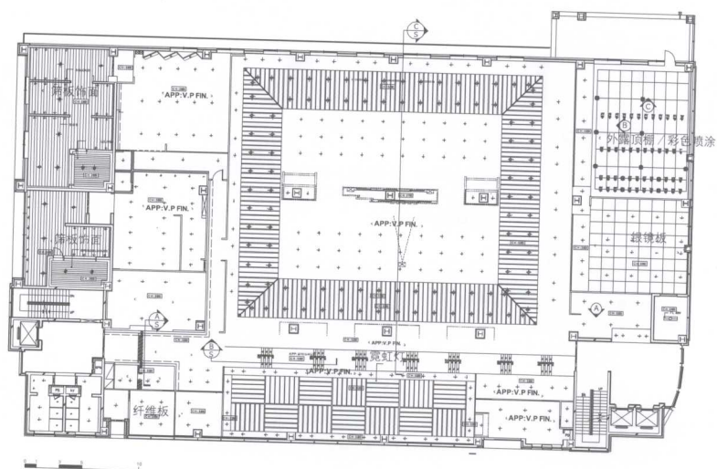
顶棚平面
