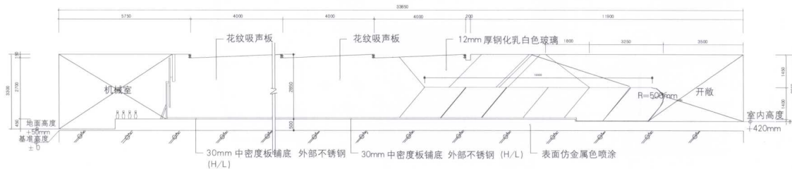
立面图 B
