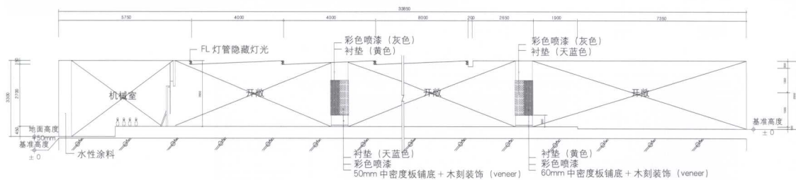
立面图 A
