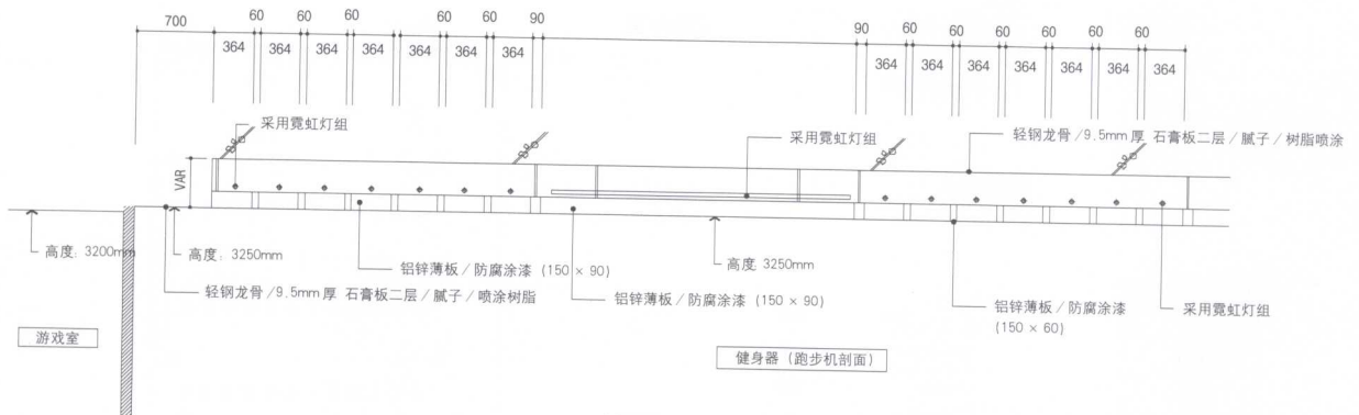
剖面图 B
