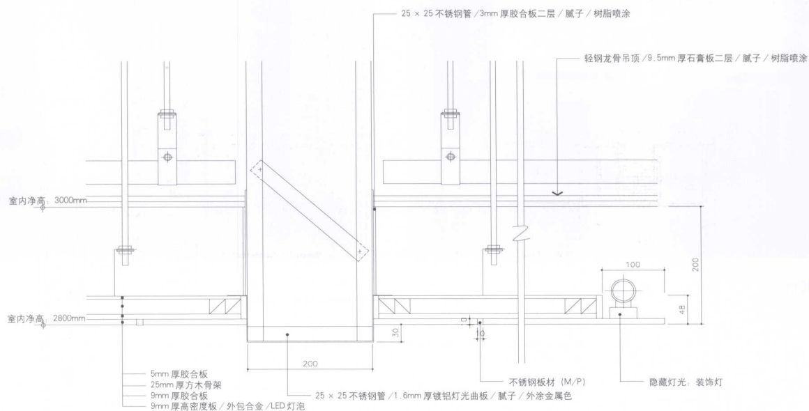
吧台一顶棚剖面细部图 A
