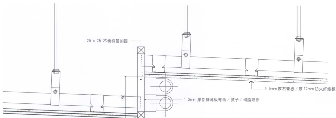
顶棚局部剖面图 B
