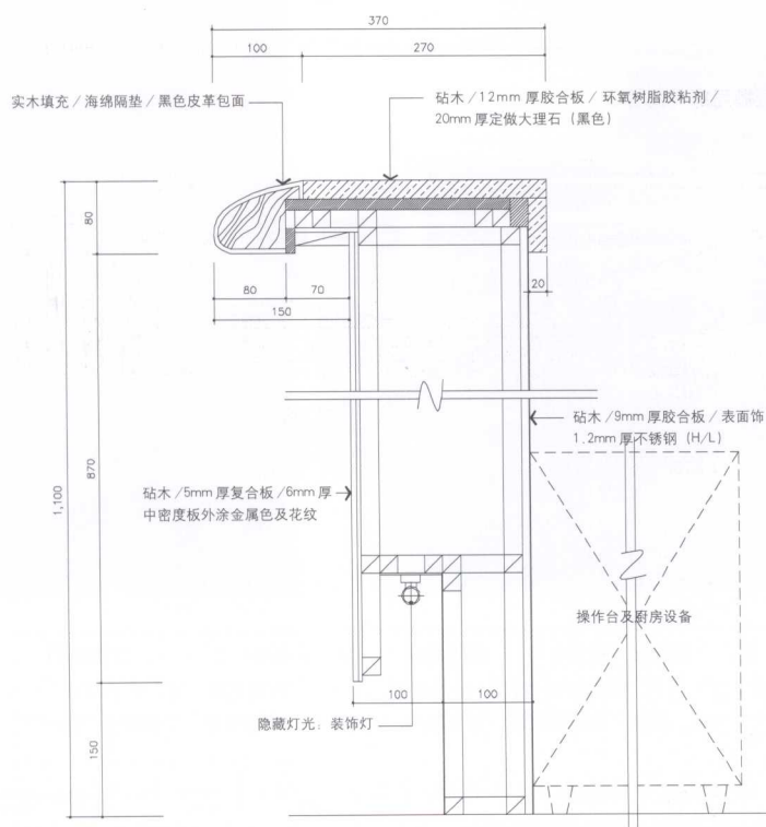
吧台桌剖面图及细部图 A'
