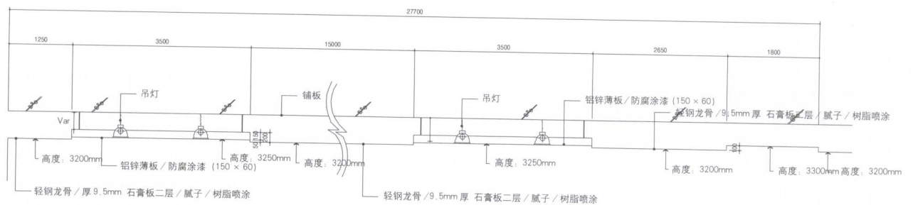
剖面图 C
