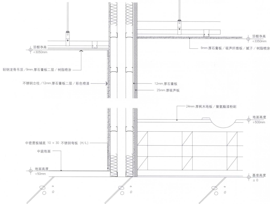
墙一剖面图及细部图 E'
