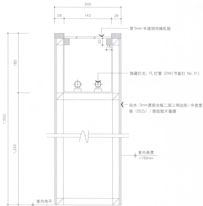
局部详图一剖面图 B'、C'
