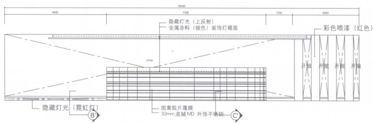
立面图 C、D
