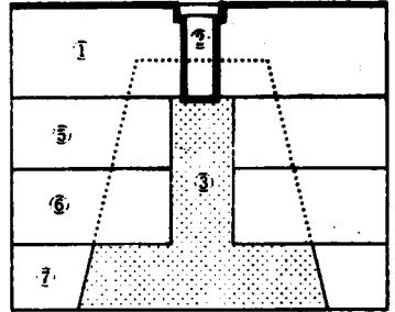
普陀峪定陵地宫金井
