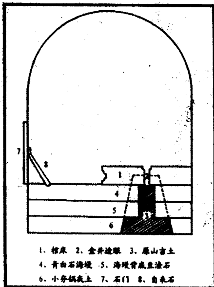
慈禧陵地宫金井示意图 (天津大学王其亨教授绘制)
