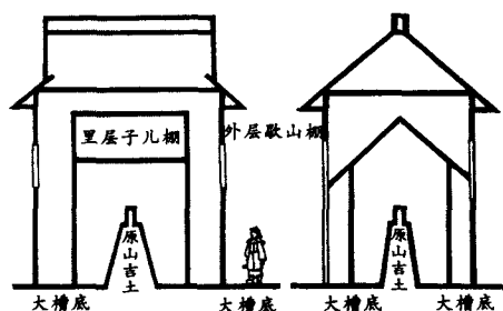
吉土罩棚剖面图 (天津大学王其亨教授绘图)
