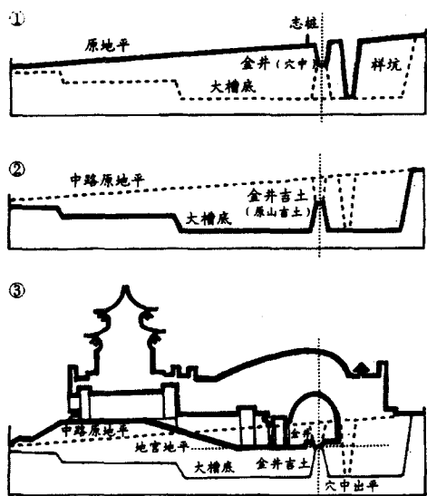
吉土罩棚剖面图 (天津大学王其亨教授绘图)
