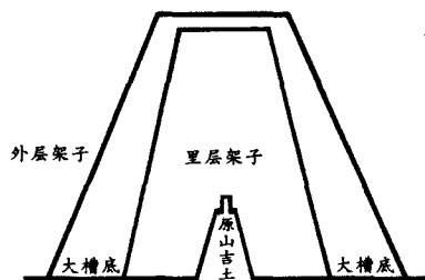
保护吉土架子剖面图 (天津大学王其亨教授绘图)
