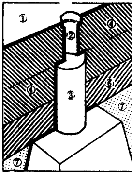
景陵土金井构造剖切透视
