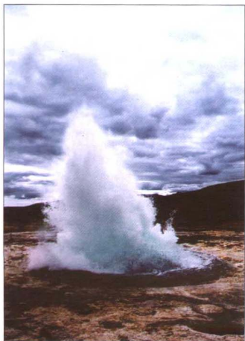
盖锡尔大间歇喷泉
