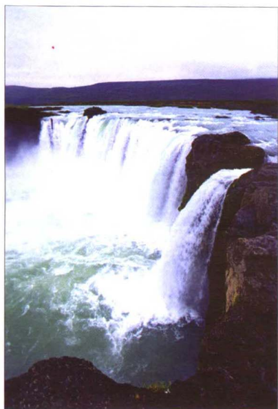
欧洲水量最大的代蒂瀑布
