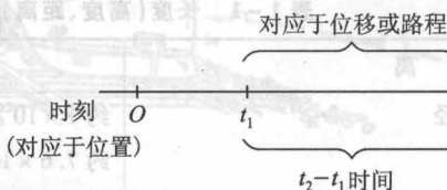
图 1-4 时间与时刻在数轴上的表示
