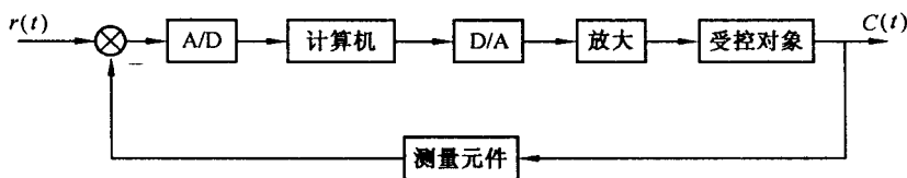
图 1.8 典型计算机控制系统框图
