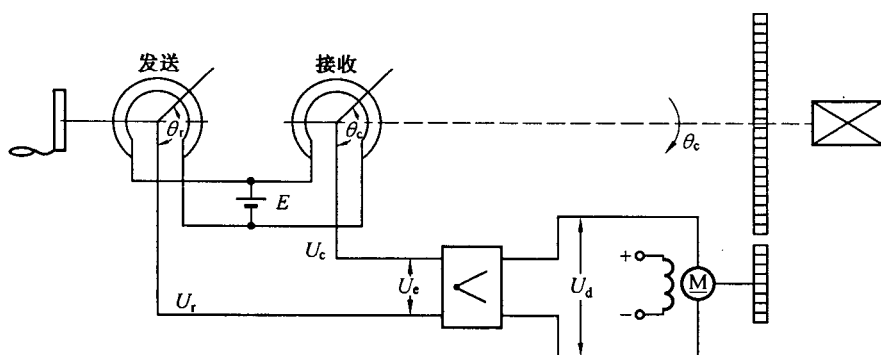
图 1.7 位置随动系统
