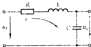
图 2.1 R-L-C 电路
