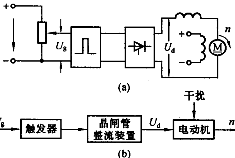
图 1.2 开环直流调速系统
