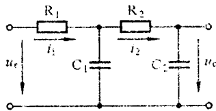
图 2.2 RC 滤波电路
