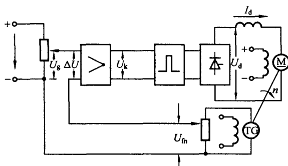
图 1.4 闭环直流调速系统
