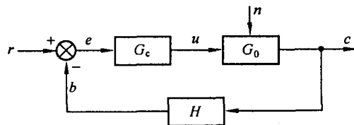
图 1.5 典型反馈控制系统
