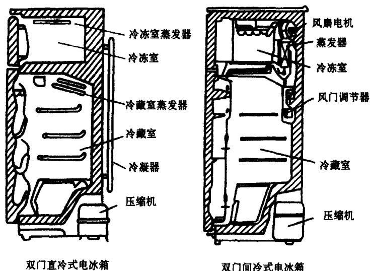
图 1-1 双门电冰箱的基本结构
