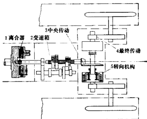
图 2-2 履带拖拉机传动系组成
