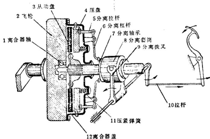
图 2-3 摩擦式离合器作用原理简图
