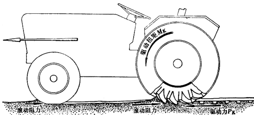
图 1-3 轮式拖拉机的工作原理
