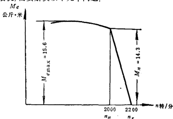
图 1-5 490 柴油机的调速特性
