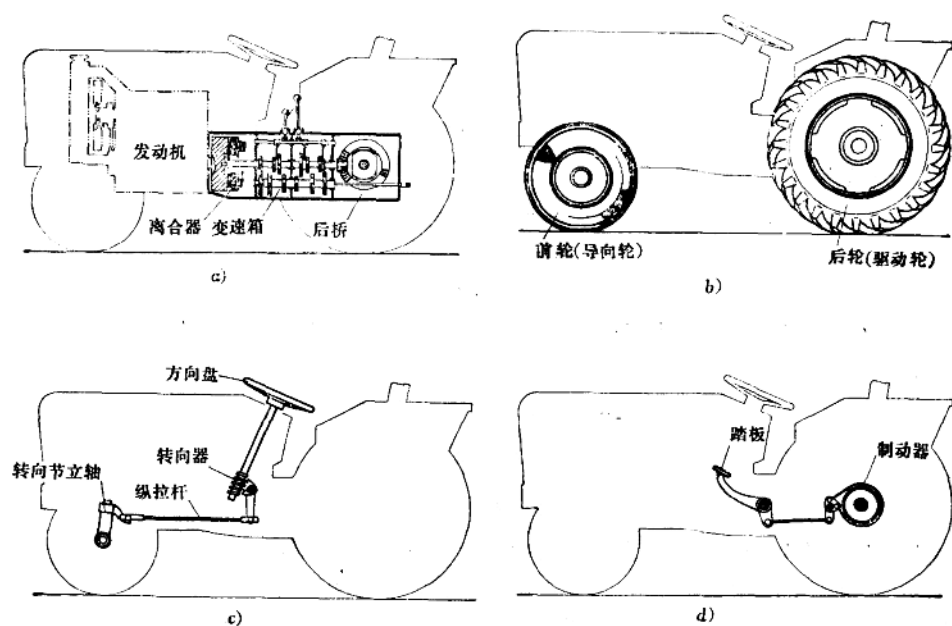
图 1-1 轮式拖拉机底盘
