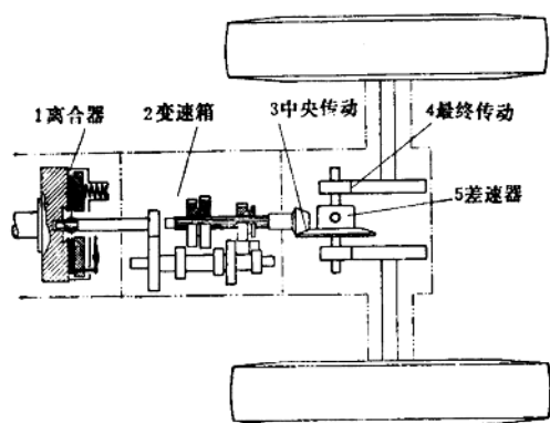
图 2-1 轮式拖拉机传动系组成
